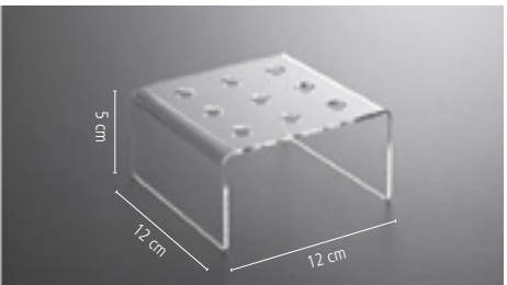
HA101 SOPORTE PLÁSTICO CUADRADO (9 mini conos) PLASTIC HOLDER SQUARE (9 mini cones) • 8u
