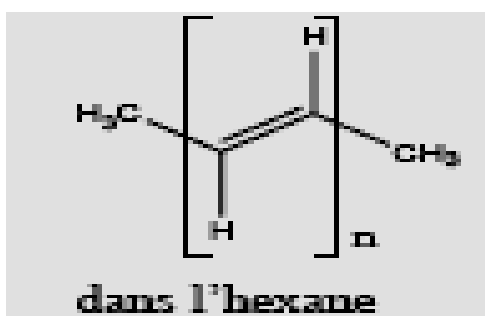
Evolution de \lambda et de \epsilon et avec la conjugaison
