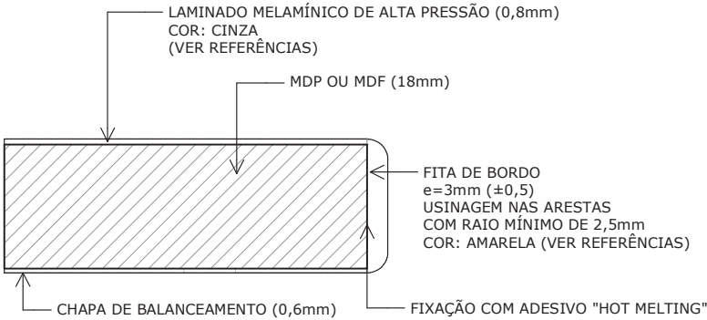
DETALHE 2 ESC. 1 : 1
